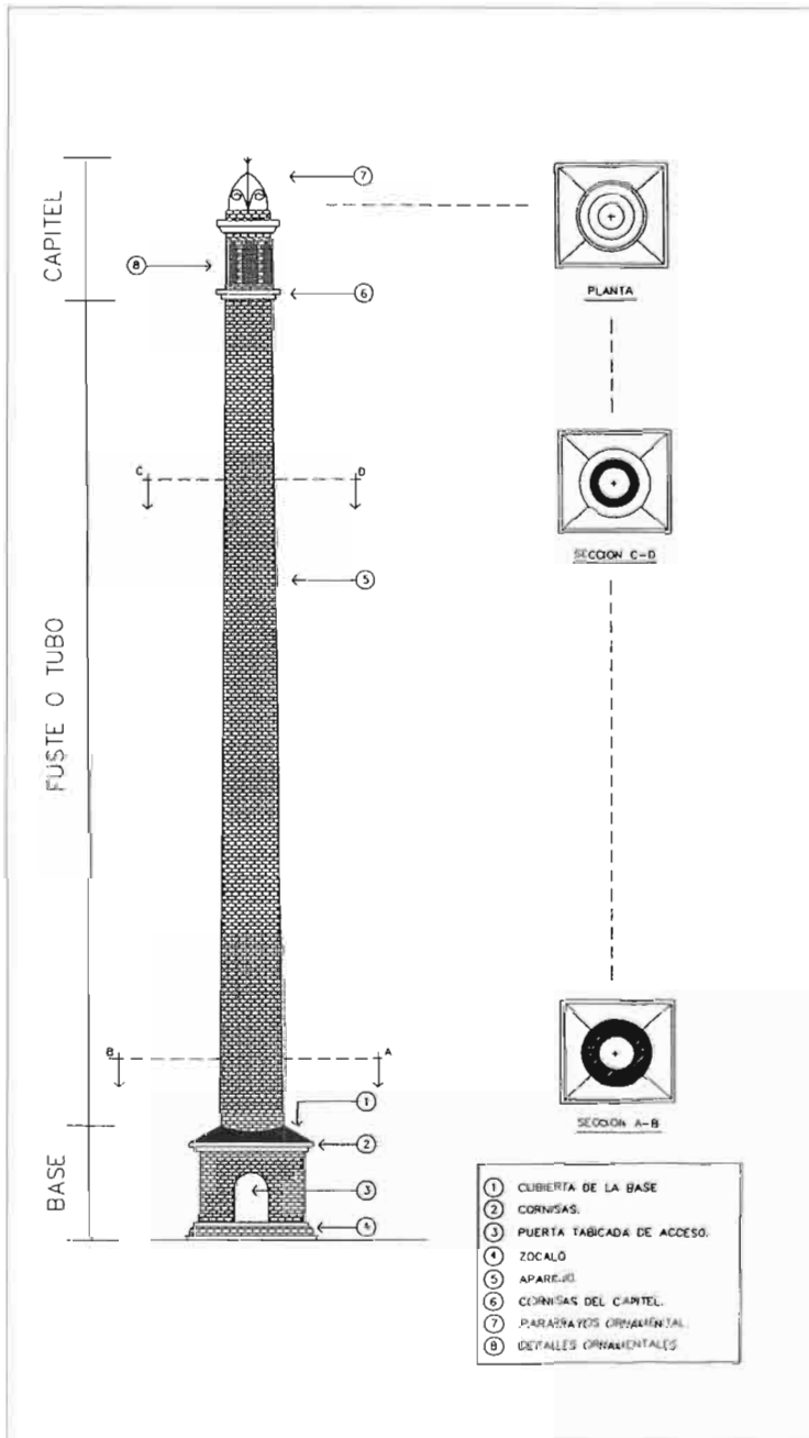
Fot. 1 .- Dibujos de una chimenea industrial. Tomado de BARACE, A y RUEDA, A., Chimeneas industriales de ladrillo . Proyecto final de carrera de la Escuela de Arquitectura Técnica de Barcelona. 1996.
