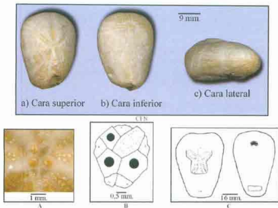
Figura 27. Cyclaster heberti CFN. A. Sistema apical; B. Sistema apical-plumilla; C. Fasciolas peripetalifera y subanal-plumilla.
