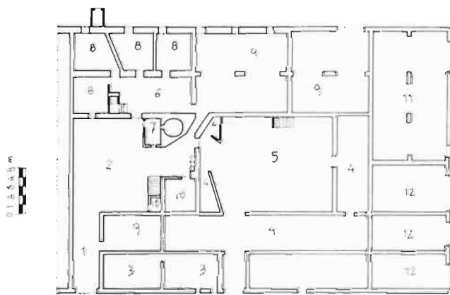
GRÁFICO 3. Planta de la "casa de los labradores" de la Casa Colorá.
