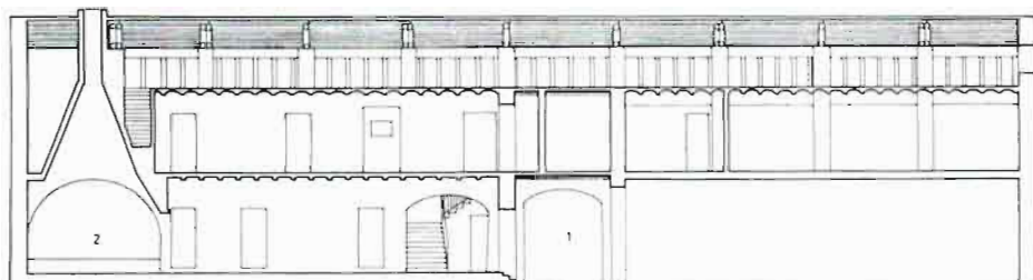
GRÁFICO 39. Sección longitudinal de la Venta del Puerto.
