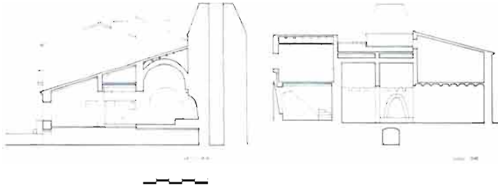
GRÁFICO 34. Secciones transversal y longitudinal del M. o de los Álamos por la sala de moler.
