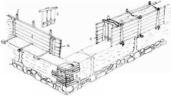
GRÁFICO 24. Construcción del tapial según A. Cámara Niño.
