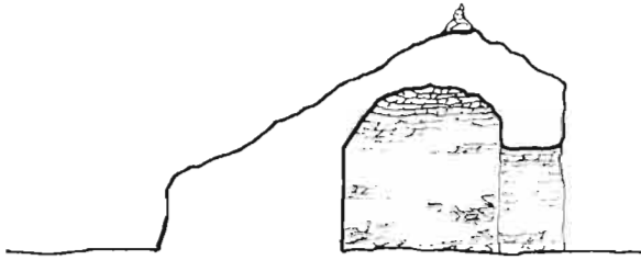
GRÁFICO 52. Sección de un Bombo según L. Feduchi.
