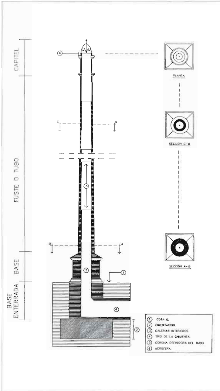
Fot. 2 .- Dibujos de una chimenea industrial. Tomado de BARACE, A y RUEDA, A., Chimeneas industriales de ladrillo . Proyecto final de carrera de la Escuela de Arquitectura Técnica de Barcelona, 1996.
