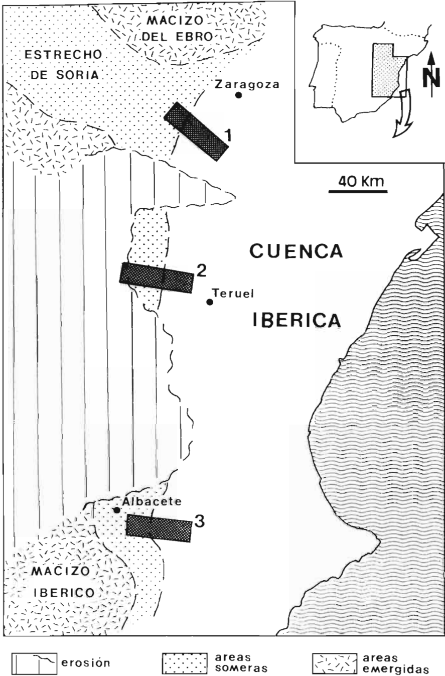
Fig. 1. Esquema paleogeográfico de la cuenca Ibérica durante el Kimmeridgiense, en el que se muestra la localización del sector estudiado (sector 3) y de los sectores septentrionales con los que se compara (sectores 1 y 2).
