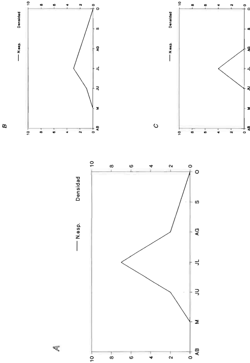
Fig. 8: Evolución estacional del número de especies y su abundancia (densidad) en el conjunto de los biotopos estudiados, correspondiente a las comunidades herbáceas. Se representan independientemente los datos correspondientes al conjunto de los necrópteros (A), y a las familias Myrmeleontidae (B) y Ascalaphidae (C).
