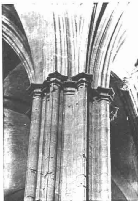
Figura 9.- Pilar exento. S. Blas. Villarrobledo.
