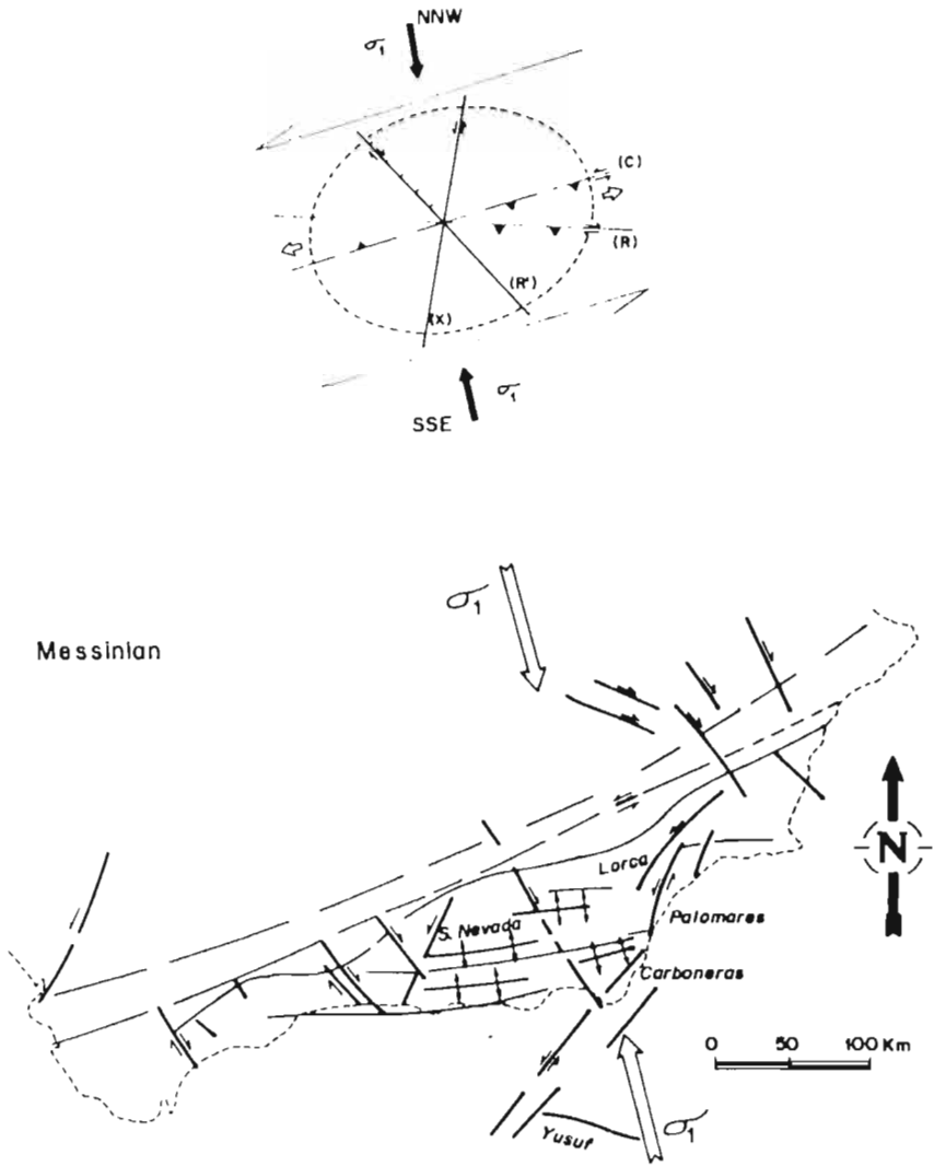
Fig. 57: Situación tensional en las Cordilleras Béticas durante el Messiniense (según Sanz de Galdeano, 1990, ligeramente modificado).
